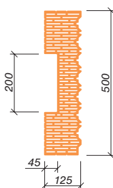
Porotherm 50 EKO+ Profi 1/2 K (1/2 K = polovičná koncová)
