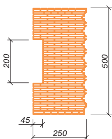
Porotherm 50 EKO+ Profi K (K = koncová)
