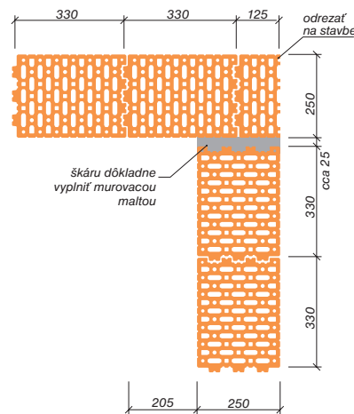
Dvojitá stena hr. 540 mm
