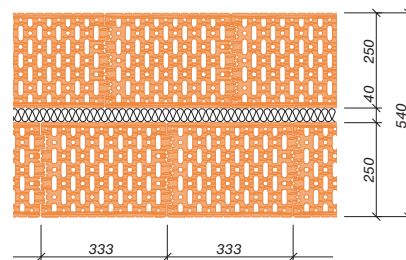
Dvojitá stena hr. 540 mm
