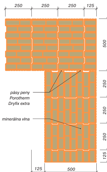
Väzba rohov a ostení
