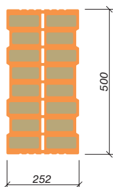
Porotherm 50 T Profi Dryfix 1/2 (1/2 = polovičná)
