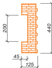
Porotherm 38 Ti Profi 1/2 K (1/2 K = polovičná koncová)
