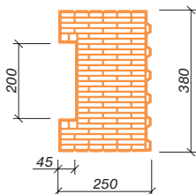
Porotherm 38 Ti Profi K (K = koncová)
