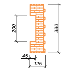
Porotherm 38 KOMBI Profi 1/2 K (1/2 K = polovičná koncová)
