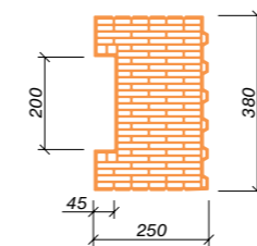
Porotherm 38 KOMBI Profi K (K = koncová)
